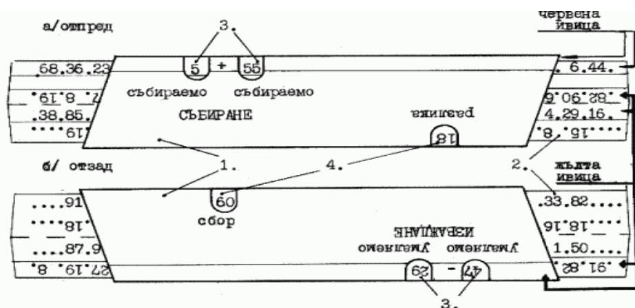
Рис. 1. Макет саморобного калькулятора
