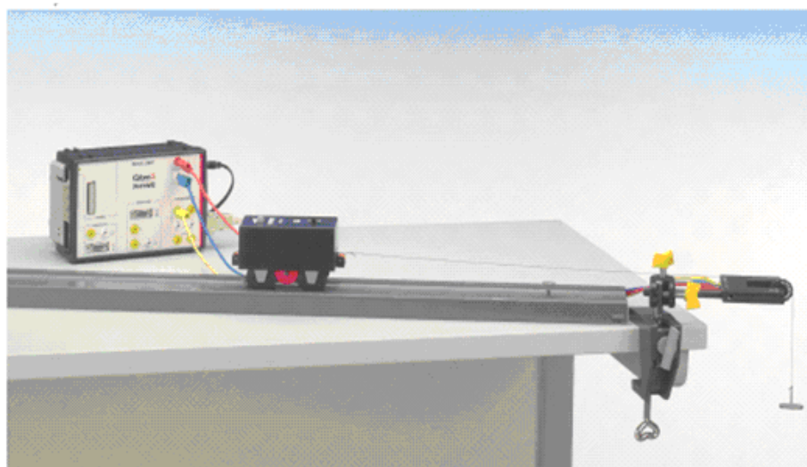
Рис. 2. Приклад комп'ютерно-орієнтованої навчальної лабораторної установки
