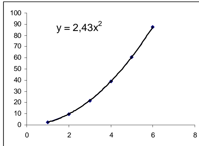
Рис.6. Графік залежності пройденого шляху від часу
