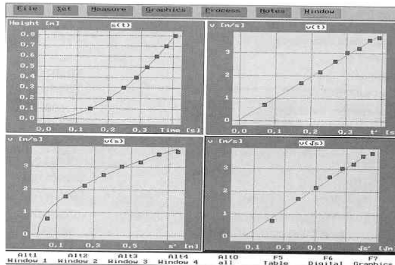
Рис. 3. Приклад образу, отриманого при навчальному дослідженні рівноприскореного руху
