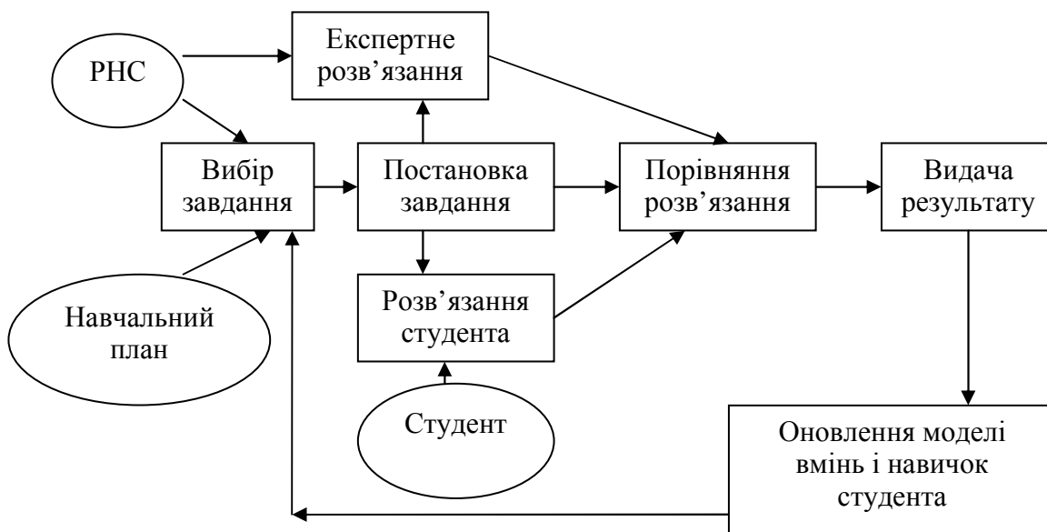
Рис. 1. Схема процесу роботи ІНС
